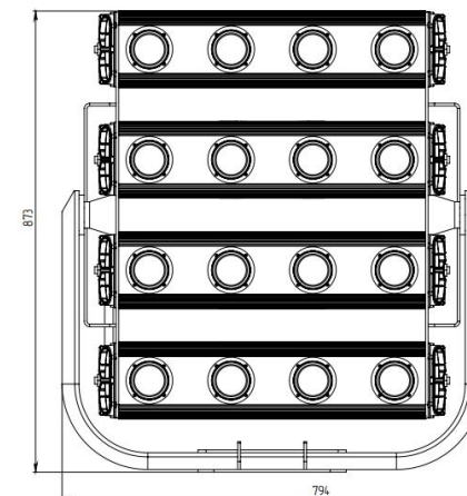
Рисунок 2. Габаритный чертеж
